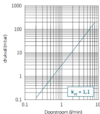
Drukverlies diagram:
